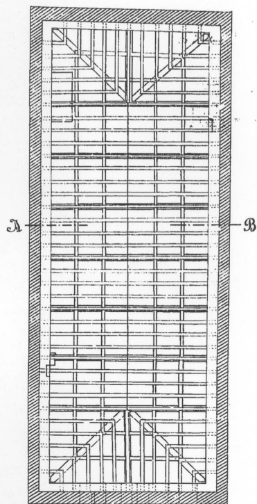
- Plattegrond Bestaande Bekapping.
