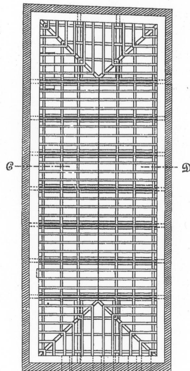
Plattegrond - Nieuwe Bekapping.
