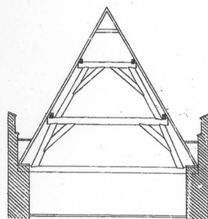
Doorsnede over A. B.
