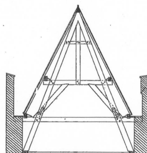
Doorsnede over C. D.
